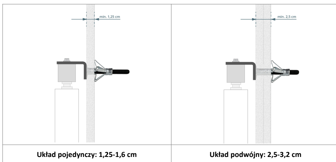
Ściana kartonowo-gipsowa - układ płyt:
